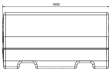
Vorderansicht
