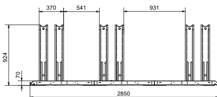
Vorderansicht
