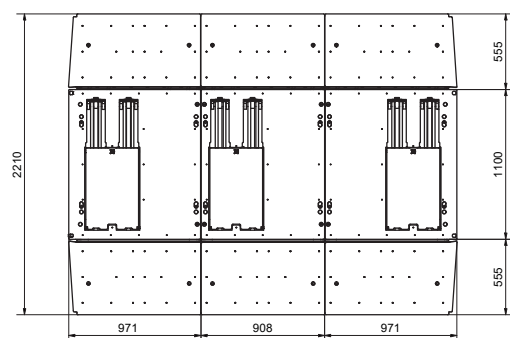
Draufsicht
