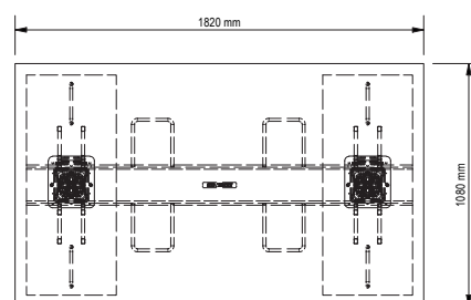
Draufsicht
