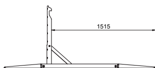
Seitenansicht
