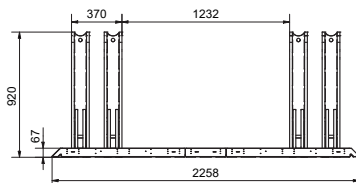
Vorderansicht
