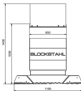
Vorderansicht
